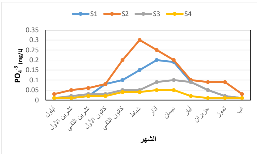
الشكل (8): التغيرات الشهرية للفوسفات في مياه نهر سوريث
