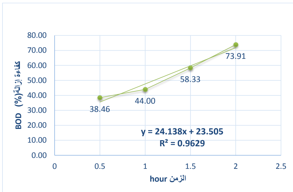
الشكل (4) العلاقة بين زمن المكث الهيدروليكي وكفاءة إزالة BOD 5
