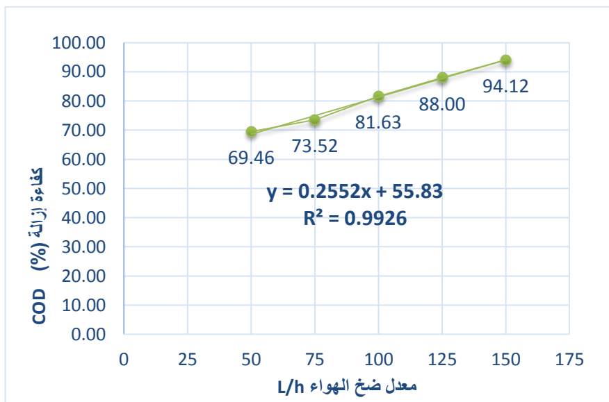
الشكل (9) العلاقة بين معدل ضخ الهواء وكفاءة إزالة COD
