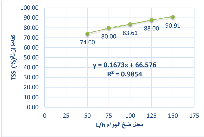
الشكل (10) العلاقة بين معدل ضخ الهواء وكفاءة إزالة TSS
