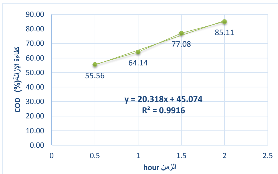
الشكل (5) العلاقة بين زمن المكث الهيدروليكي وكفاءة إزالة COD
