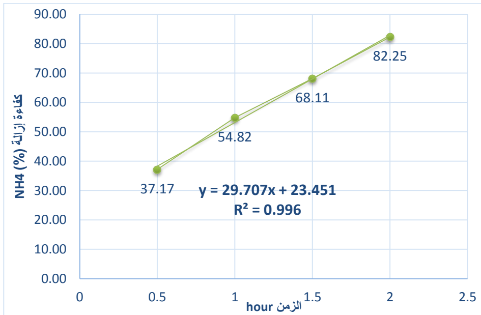
الشكل (7) العلاقة بين زمن المكث الهيدروليكي وكفاءة إزالة NH_4^+
