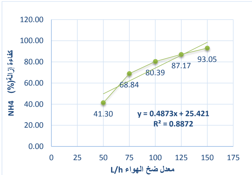
الشكل (11) العلاقة بين معدل ضخ الهواء وكفاءة إزالة NH_4^+
