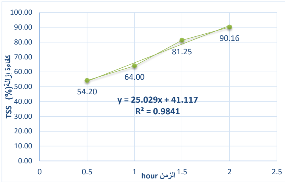
الشكل (6) العلاقة بين زمن المكث الهيدروليكي وكفاءة إزالة TSS
