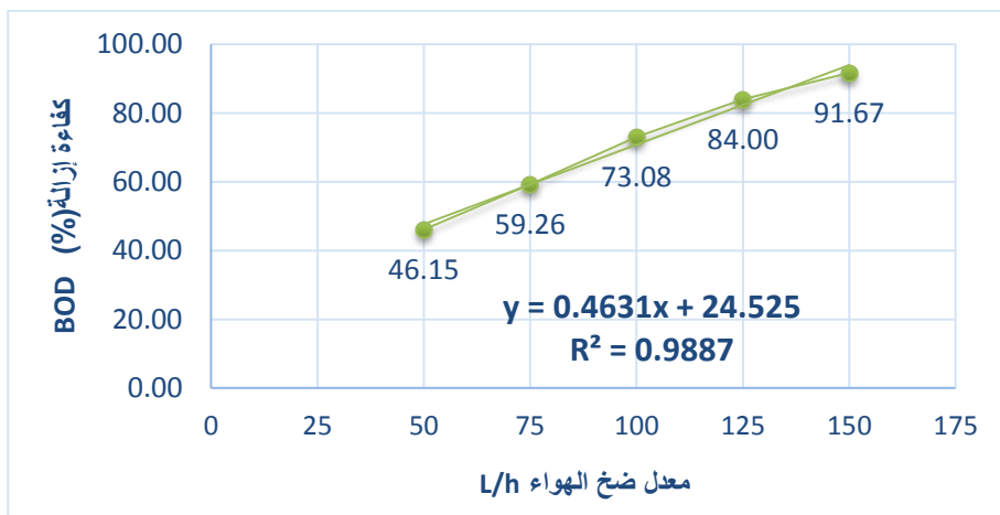
الشكل (8) العلاقة بين معدل ضخ الهواء و كفاءة إزالة BOD_5
