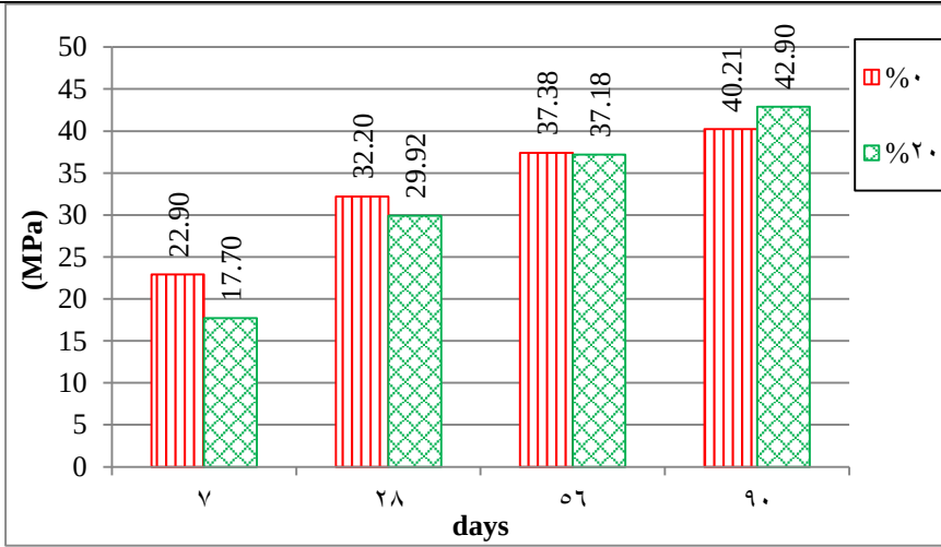
الشكل (٨) قيم مقاومة الضغط بأعمار مختلفة للعينات المرجعية والمعدلة بالتمي ٢٠%
