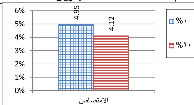
الشكل (10) قيم الامتصاص للعينات المرجعية والمعدلة بالطمي ٢٠%
