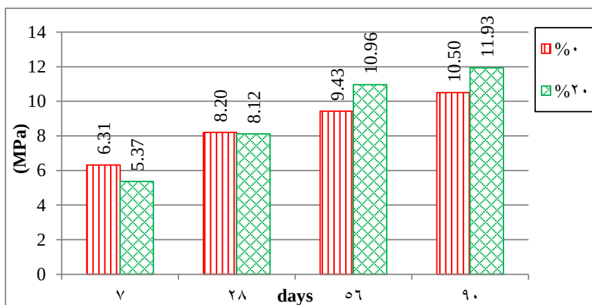
الشكل (٧) قيم مقاومة الانحناء بأعمار مختلفة للعينة المرجعية والمعدلة بالطمي ٢٠%
