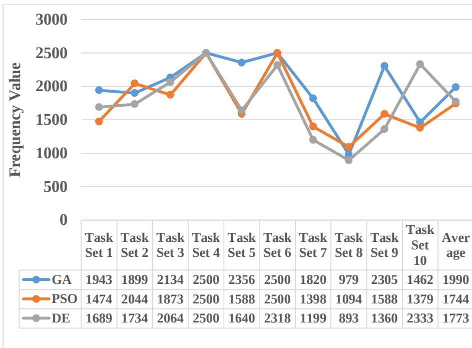
الشكل (6) مقارنة أفضل قيمة تردد عمل توصلت لها الخوارزميات التطورية المدروسة
