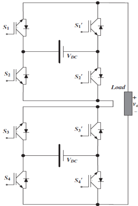
الشكل (9): دارة القدرة لإنفترت تسلسلي (CHB-MLI) ذو خمس مستويات
