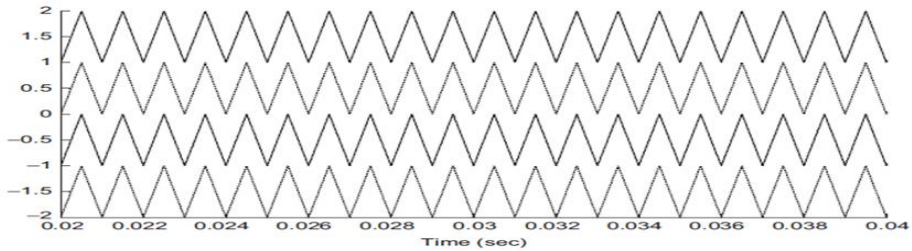
الشكل 2: استراتيجية (PD-PWM)
