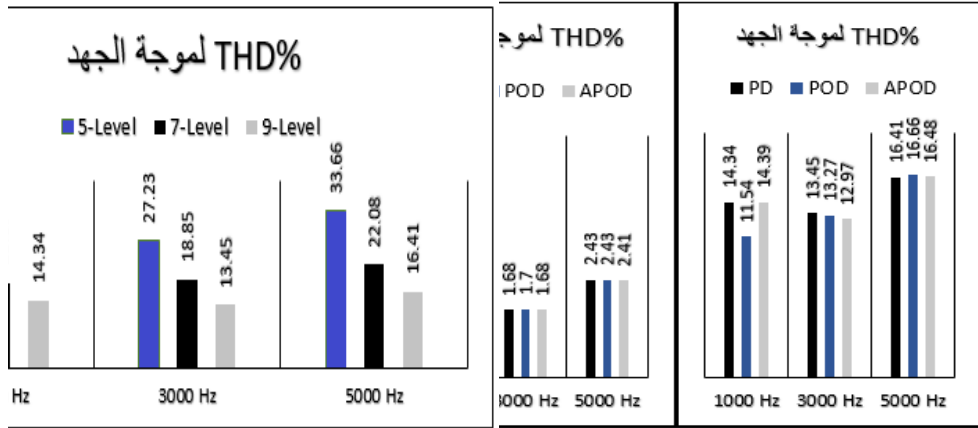
الشكل 17: معدل التشوه التوافقي عند استراتيجية PD-PWM
